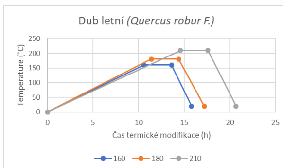
Obr. 25. Grafický průběh termické modifikace dubu letního ( Quercus robur F.)
