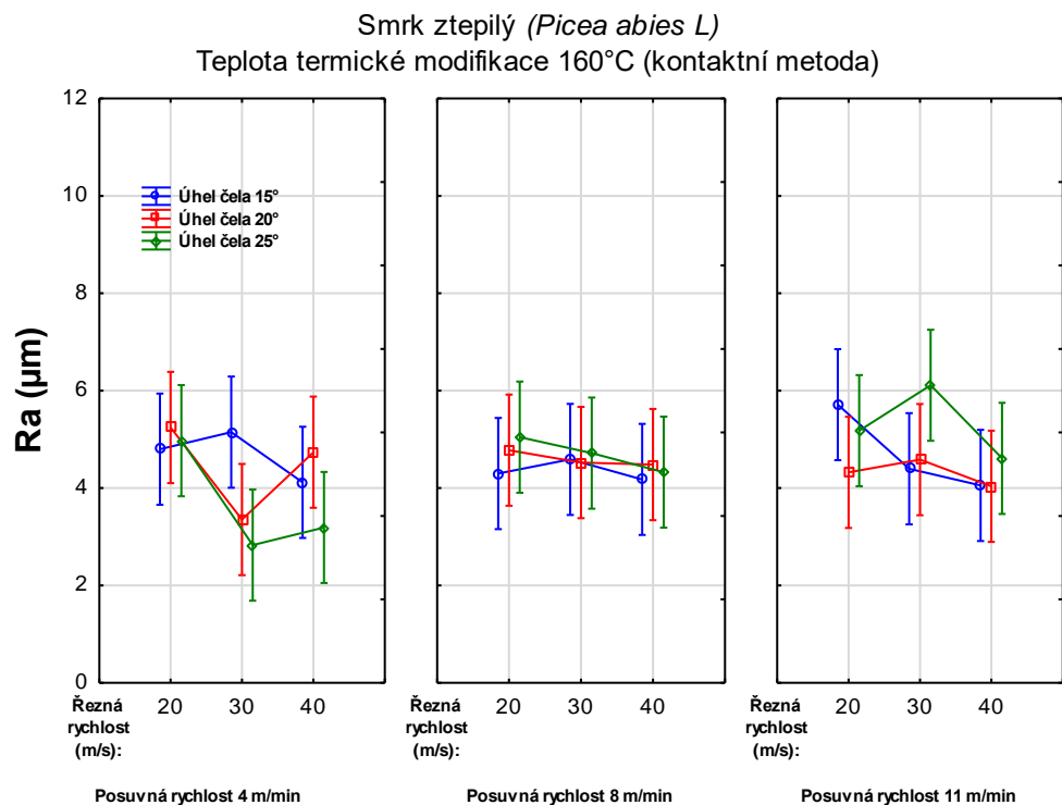
Obr. 81. Čtyř faktorová analýza drsnosti R_a termicky modifikovaného smrku na 160 °C (kontaktní metoda)
