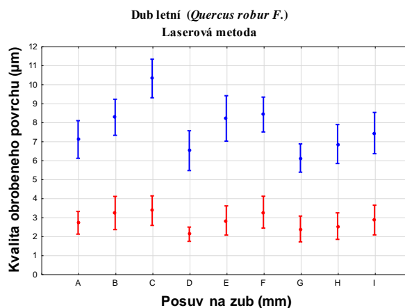
Obr. 75. Závislost vlnitosti a drsnosti povrchu na posuvu na zub, dub letní (laserová metoda)
