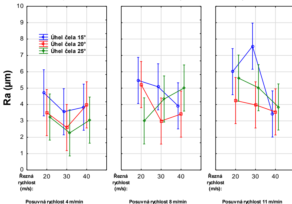
Obr. 91. Čtyř faktorová analýza drsnosti R_a termicky modifikovaného dubu na 210 °C (kontaktní metoda)
